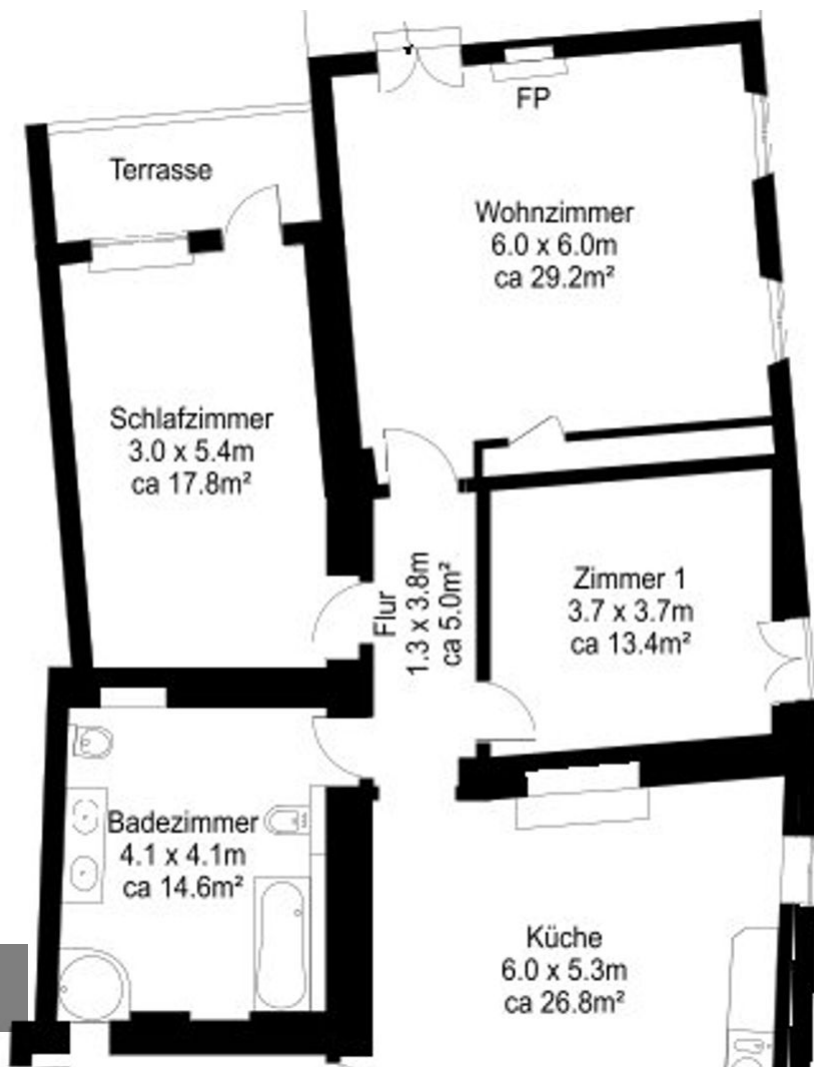
Grundrissplan EG
